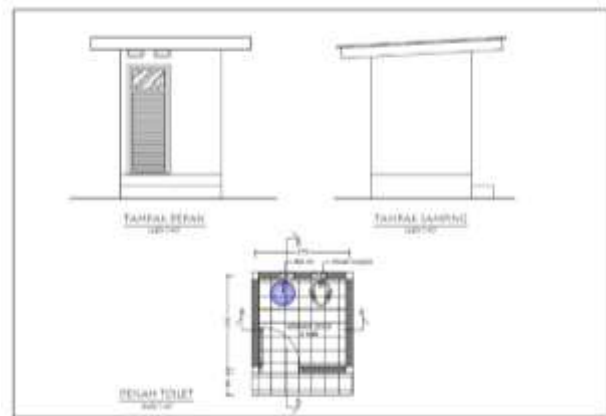
Gambar 2. (Denah Toilet yang akan dibangun di Kelurahan Ijobalit)
